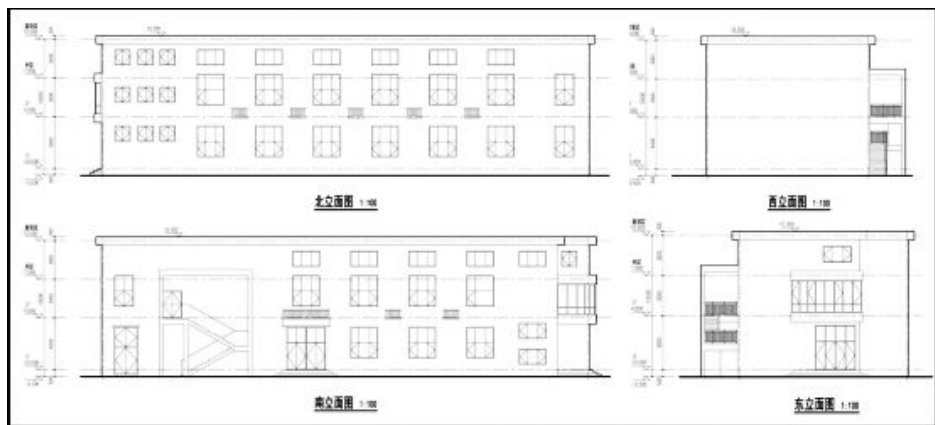
图4 建筑立面图
