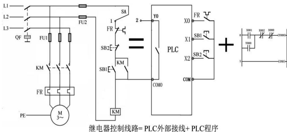
继电器控制线路=PLC外部接线+ PLC程序
